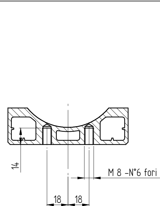
Sezione foratura
